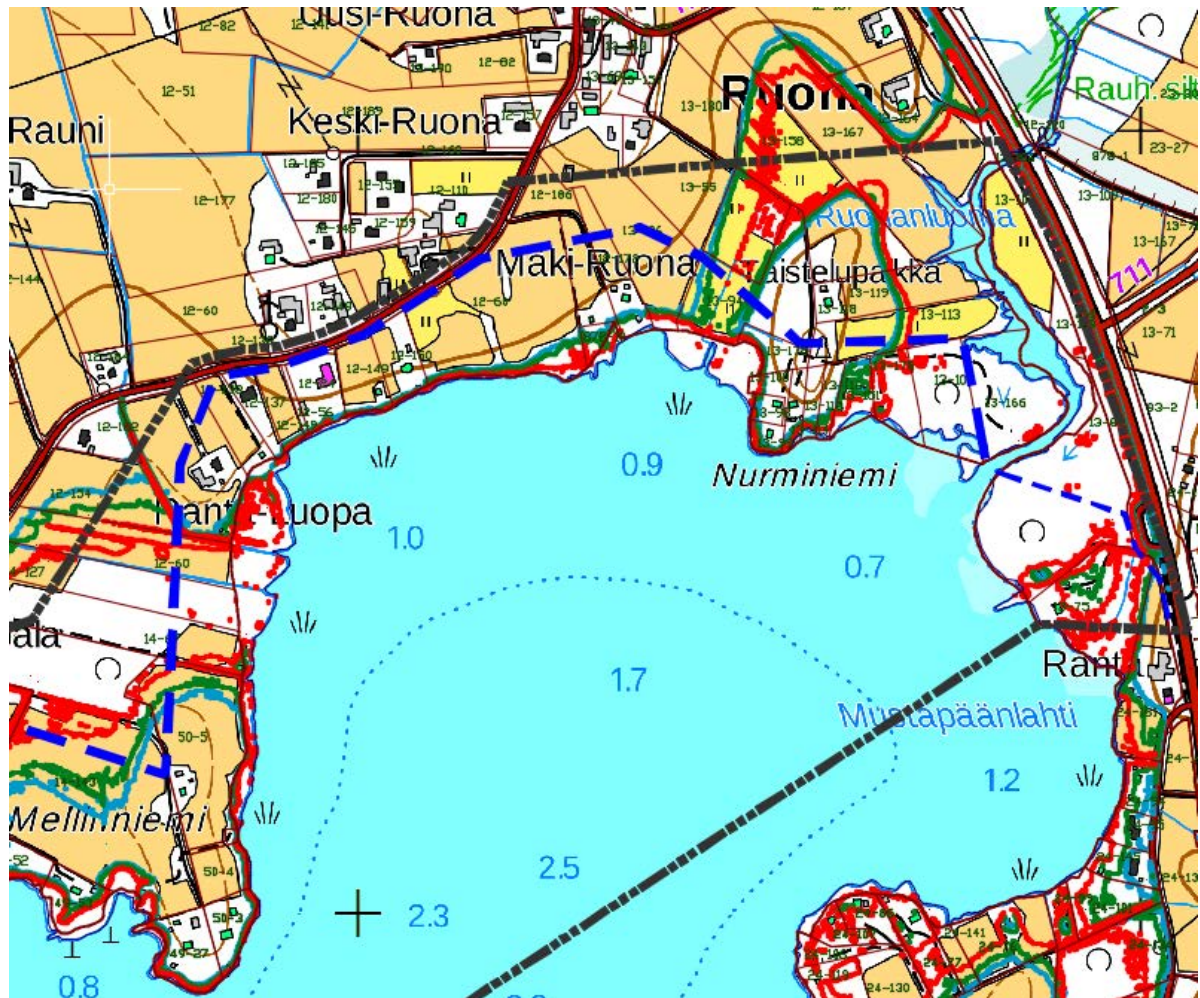
Kuva 39. Rantojen korkeusanalyysi, Ruonan alue.
