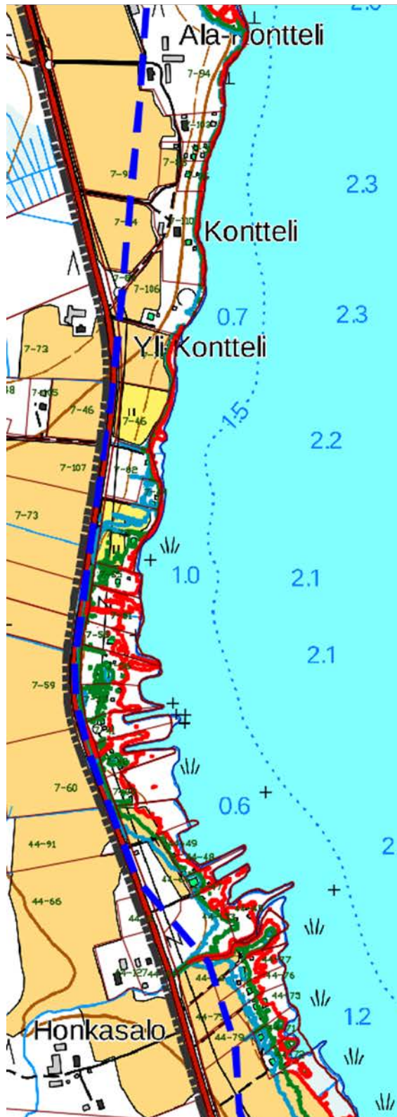
Kuva 36. Rantojen korkeusanalyysi, Länsiranta ja Maunuksen alue.
