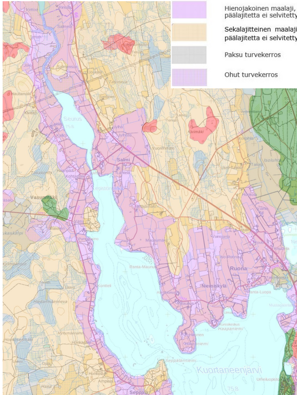
Kuva 5. Maaperäkarta 1:20 000 (Lähde GTK, Maanmittauslaitos 2019).
