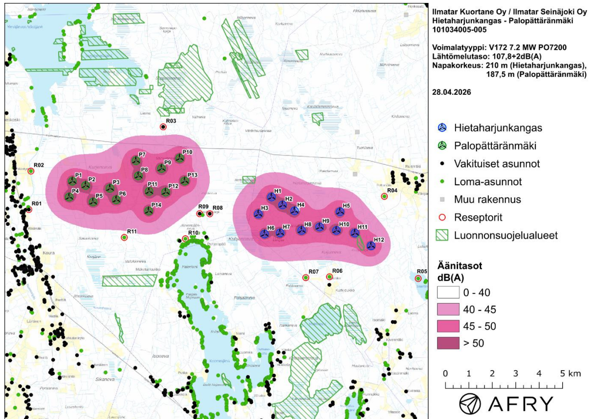
Kuva 3-2: Keskiäänitasot LAeq Hietaharjunkangas-Palopättäränmäen tuulivoimapuiston hankealueella.
