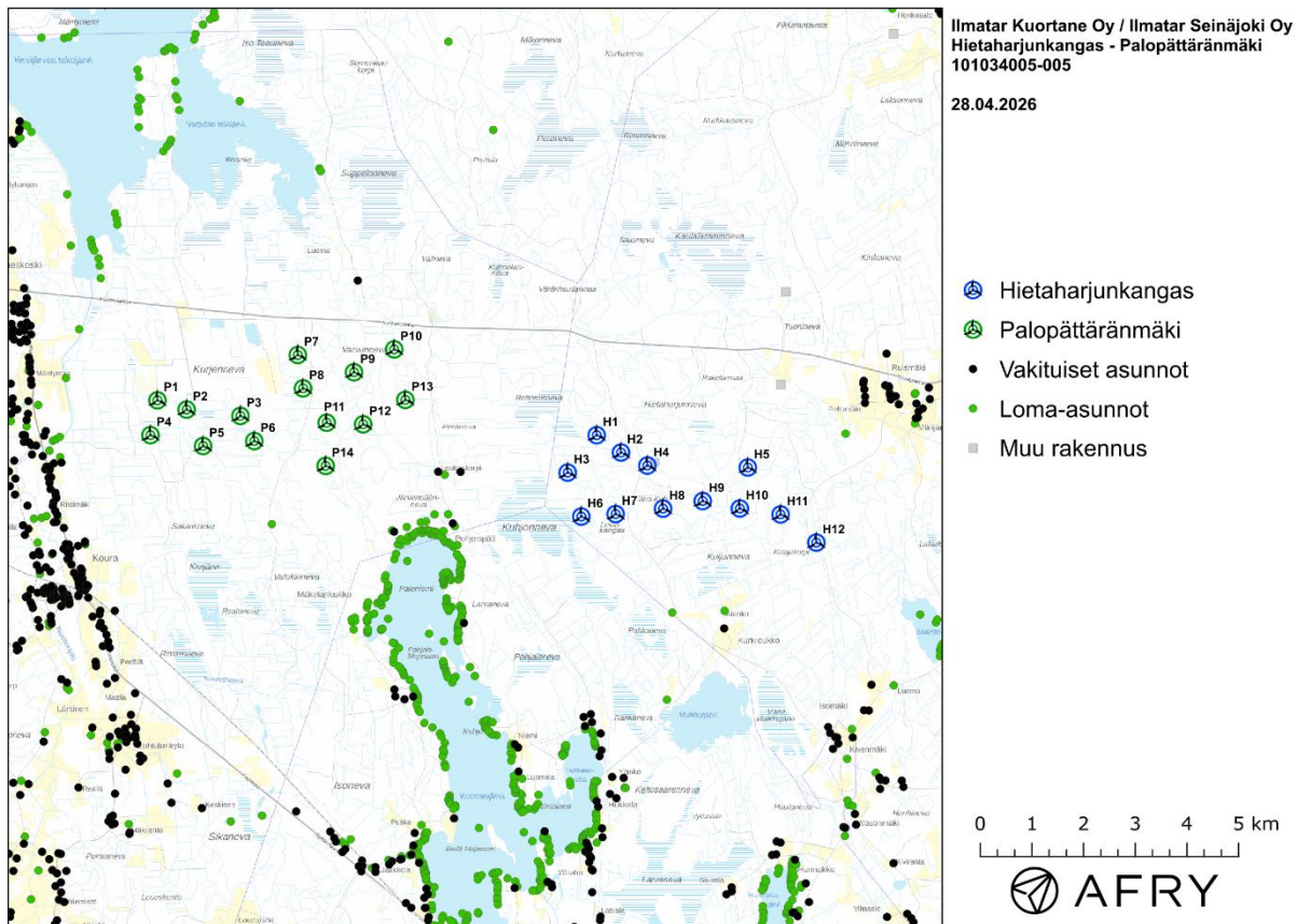
Kuva 1-1: Tuulivoimaloiden sijainnit Hietaharjunkangas-Palopättäränmäen tuulivoimapuiston hankealueella.
