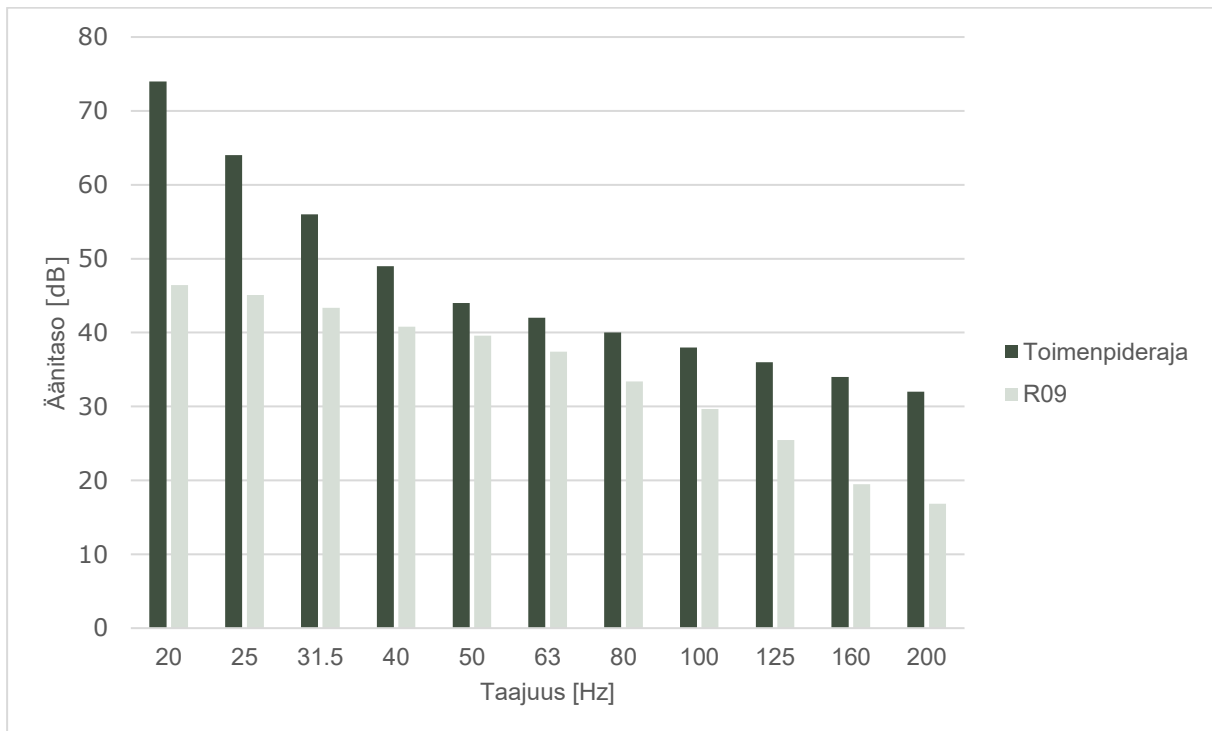
Kuva 3-3: Matalataajuisten sisämelun tasot reseptorin R09 kohdalla.
