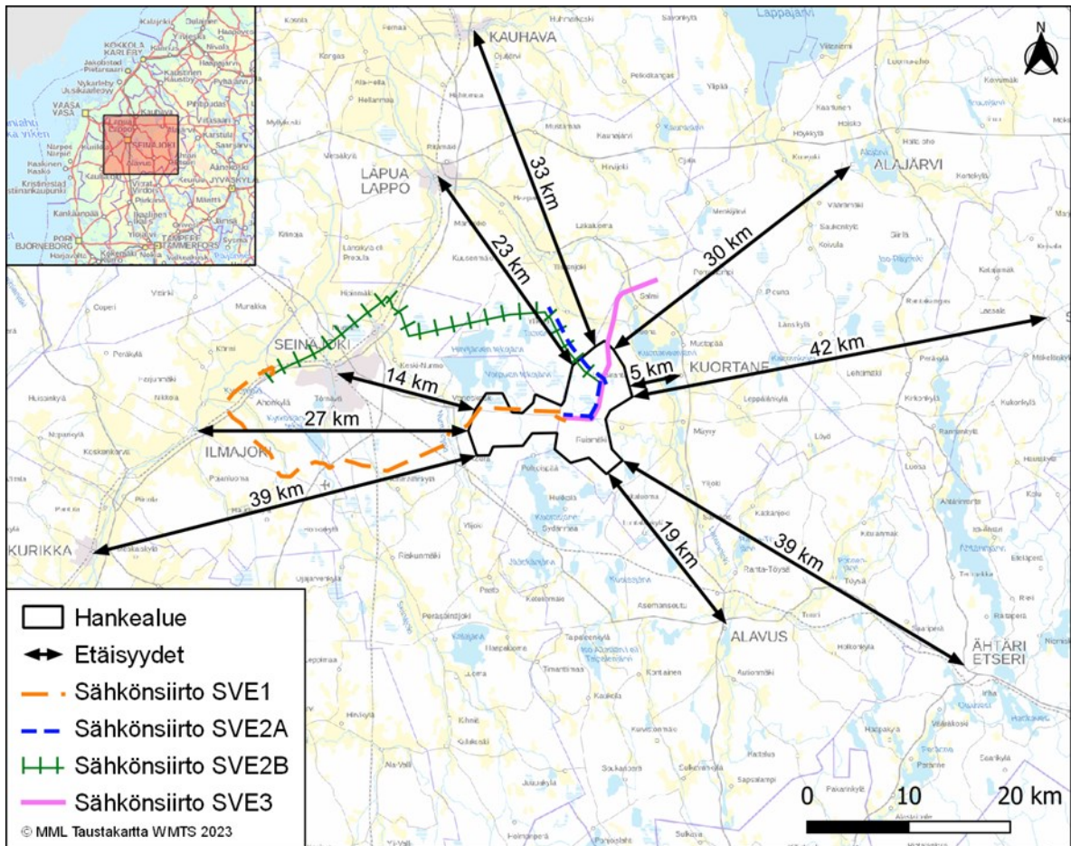
Kuva 1 Hankealueen ja sen sähkösiirtoreittien sijainti.
